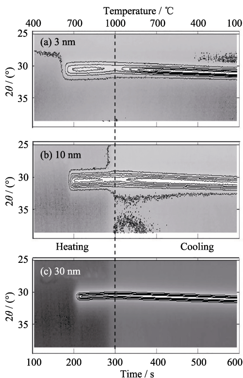
图 7 不同厚度 Si/SiO 2 /a-C/Ni(100 nm)样品在 He 气氛下加热至 1000°C 及冷却过程中原位 XRD 的(002)石墨峰强等高线图, 变温速率为 3°C/s, 厚度(a) 3 nm、(b) 10 nm 和(c) 30 nm。不同厚度 a-C 样品的等高线间隔不同 [41]
