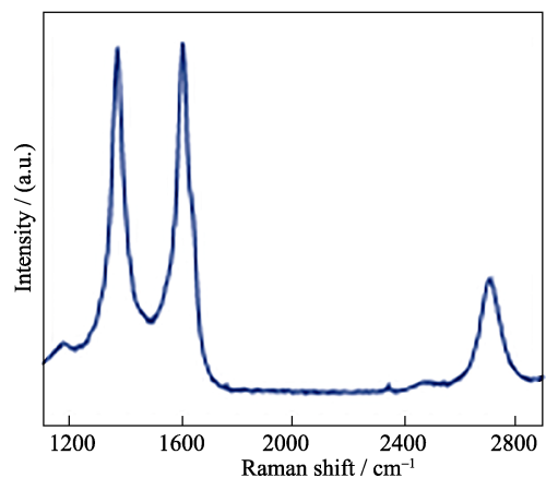
图 2 基底 200℃、氢气气氛下激光辐照样品的拉曼光谱图 [30]
