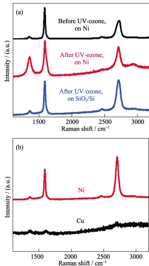
图 6 不同生长条件下拉曼分析结果 [33]
